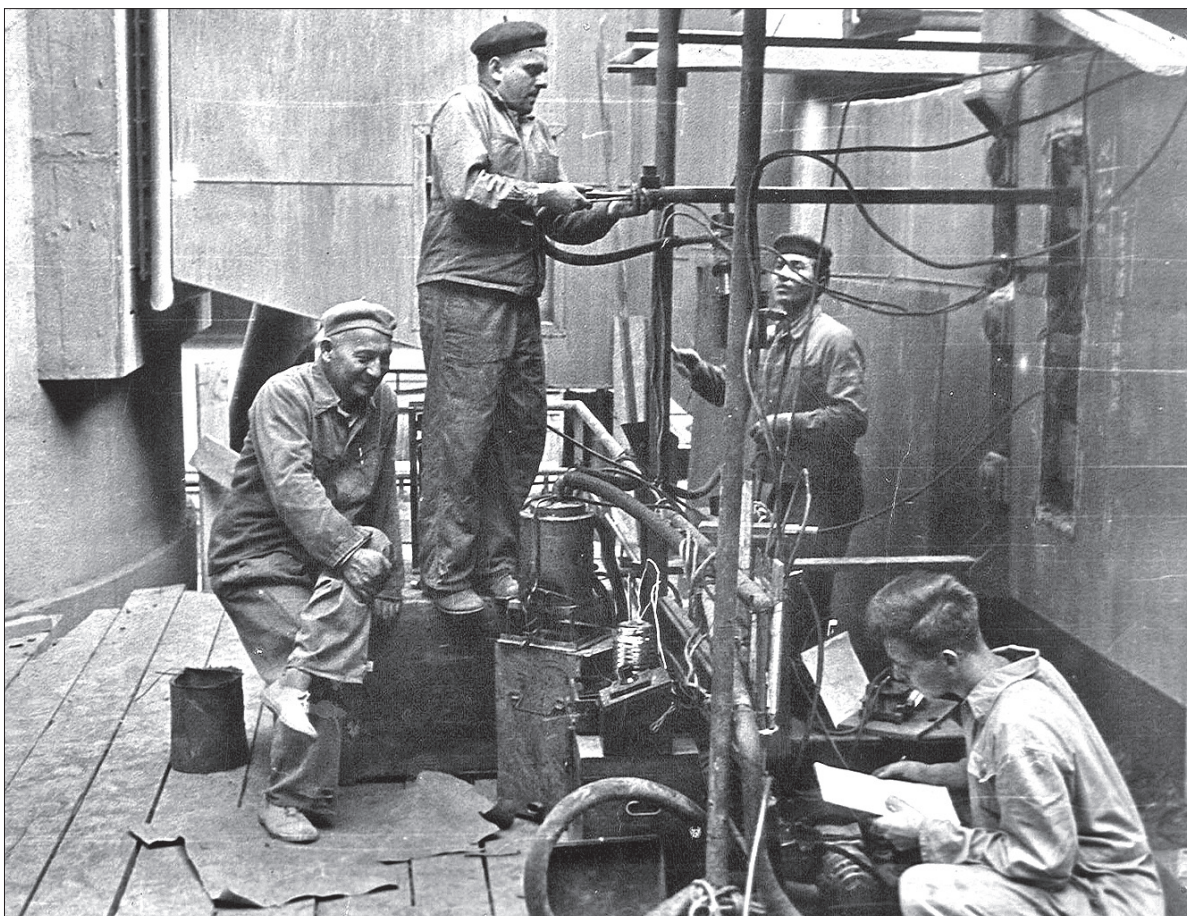
Inżynier Zygmunt Stopa podczas przeprowadzania pomiarów na kotle w elektrowni Poříčí w 1960 roku.
